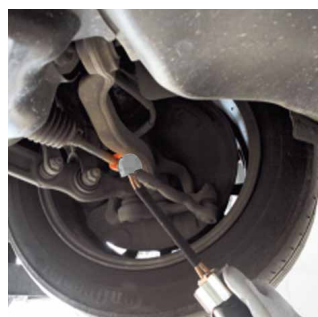
Lossar styrlänkar
